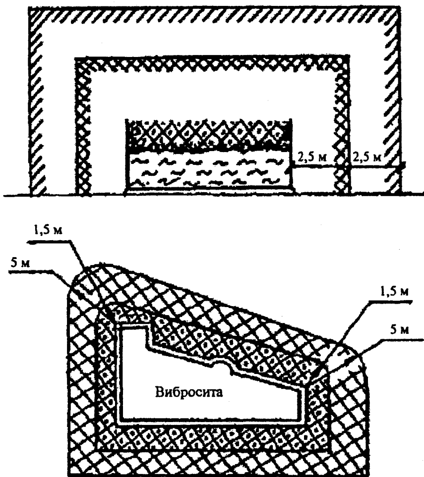
Рис. 4. Открытые пространства вокруг открытых емкостей, аппаратов, устройств
