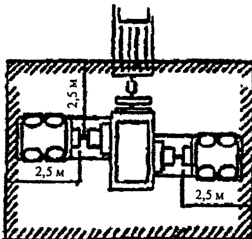
Газовый компрессор
